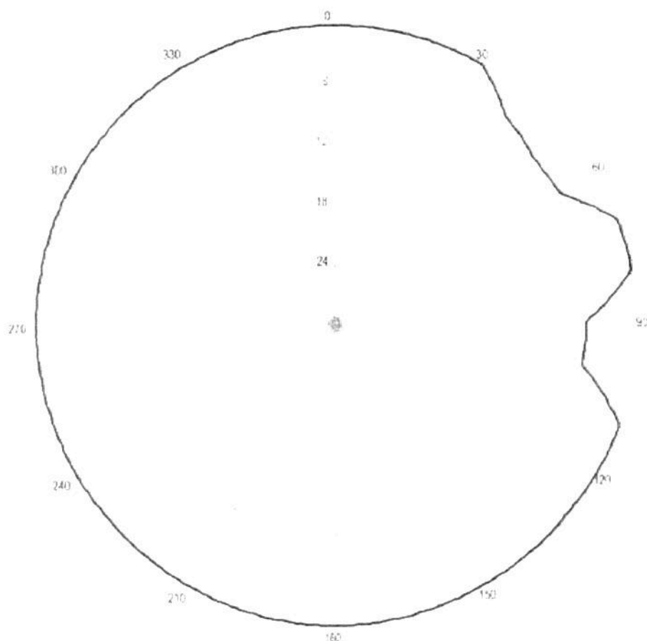
Pozioma charakterystyka promieniowania anteny stacji Września 93,7 MHz
